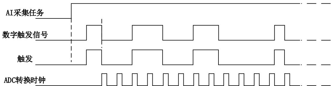
图 4-7-3 数字触发--下降沿触发
