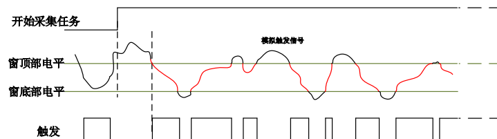
图4-8-8 模拟窗触发--入窗
