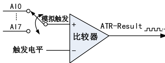
图4-8-7 比较器
