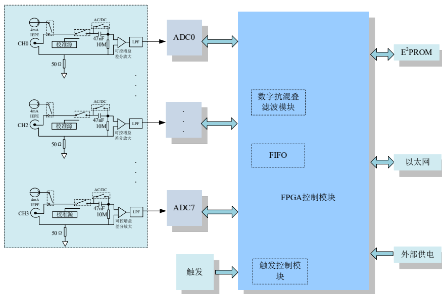
图 2.2.1 NET8814-4/8 系统框图
