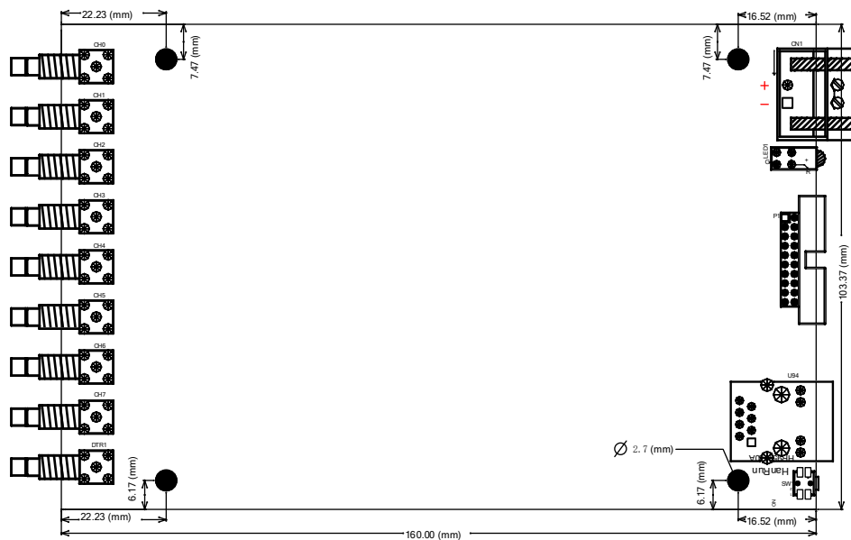
图 3-2-1 NET8814 板卡尺寸图
